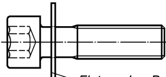
Flat washer B 5,5 DIN 6902
