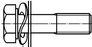
Flat washer B 5,5 DIN 6902 Curved spring washer 5,5 DIN 6904
