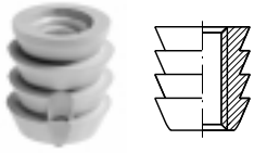
RAMPA Nylon Sockets type EM
